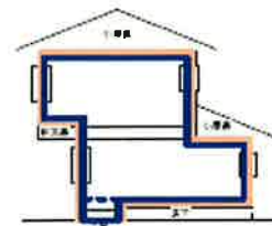
外皮平均熱貫流率 ( U_A )
